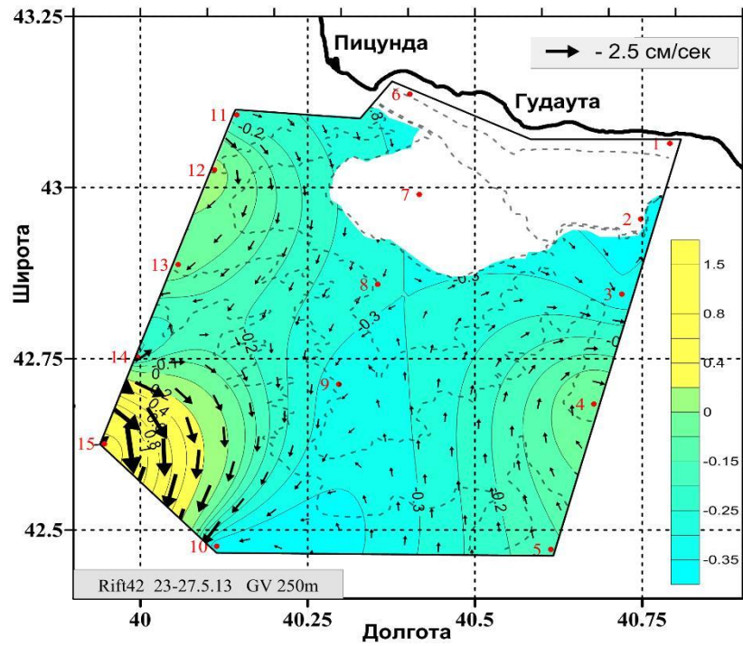
Рис. S10. Геострофические течения на горизонте 250 метров 23–27 мая 2013 г.
