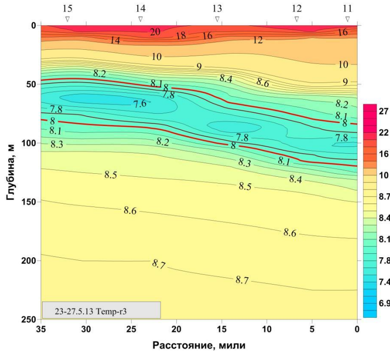
Рис. S7. Распределение по глубине температуры ( ^{\circ}\text{C} ) на разрезе 3 «берег – море» (станции 11–15). 23–27.05.2013 г. Изотермы 8^{\circ}\text{C} (красные линии) выделяют границы ХПС
