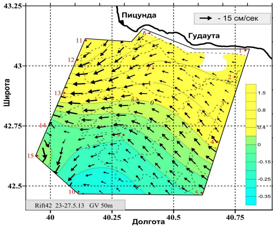
Рис. S8. Геострофические течения на горизонте 50 метров 23–27 мая 2013 г.
