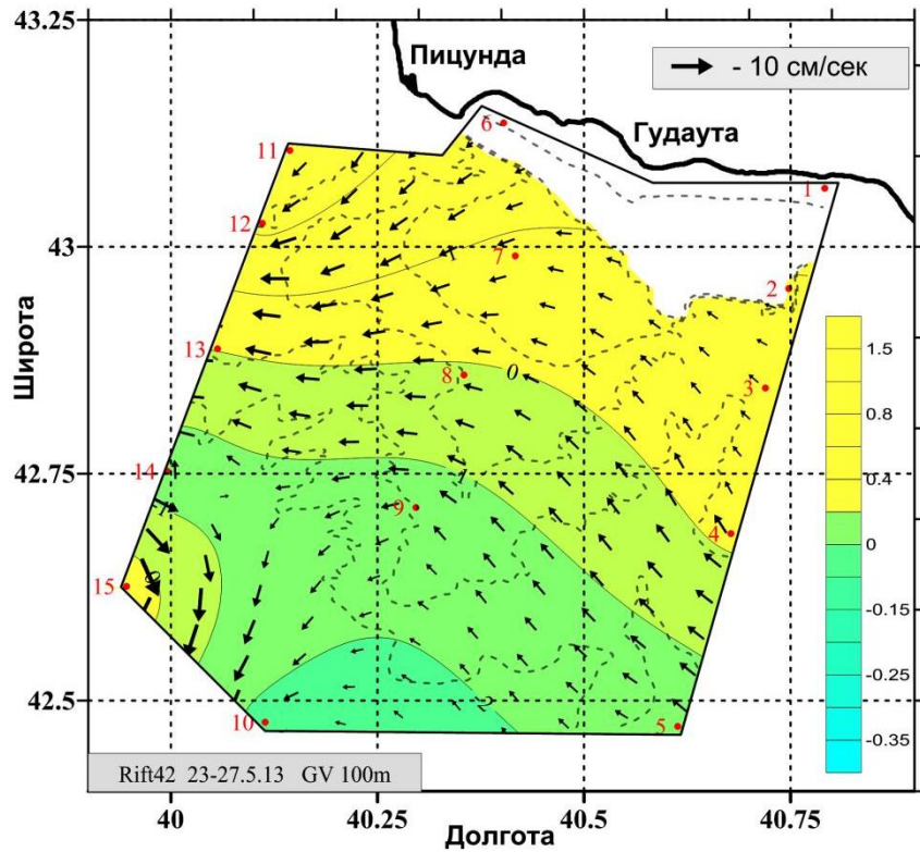
Рис. S9. Геоострофические течения на горизонте 100 метров 23–27 мая 2013 г.
