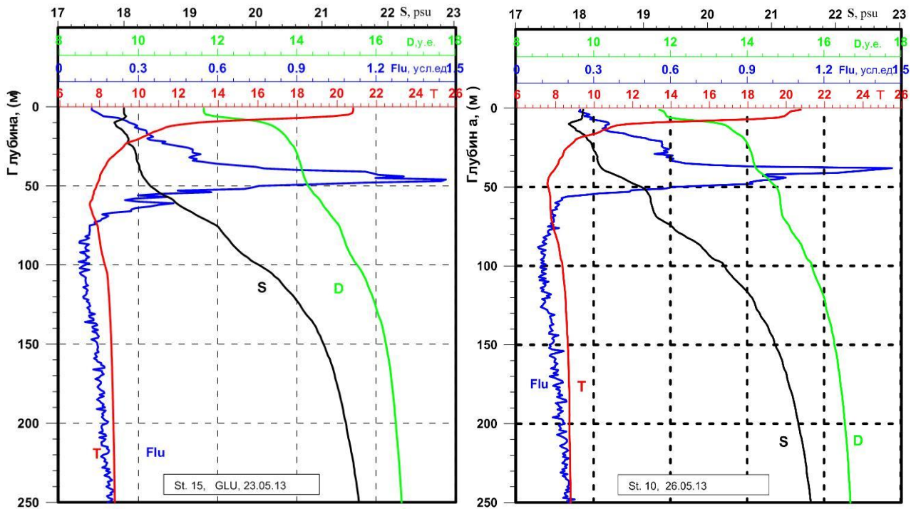
Рис. S2. Распределение с глубиной гидрологических параметров в мае 2013 г. на станциях 10 и 15.
