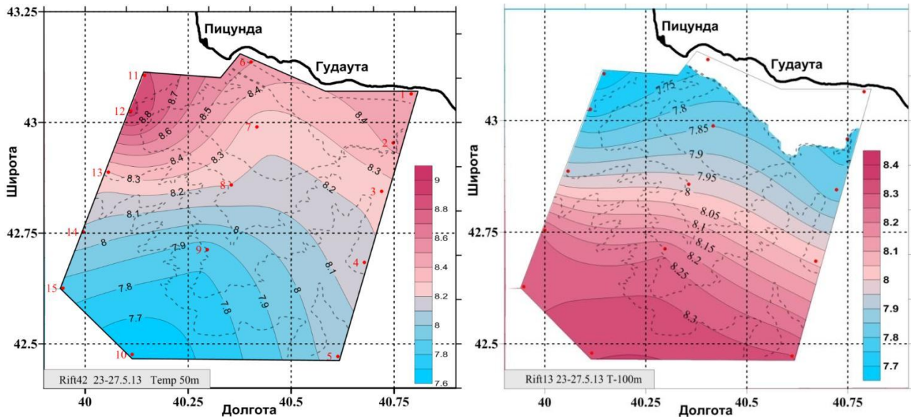
Рис. S3. Распределение температуры (°C) на горизонтах 50 и 100 метров 23–27 мая 2013 г.
